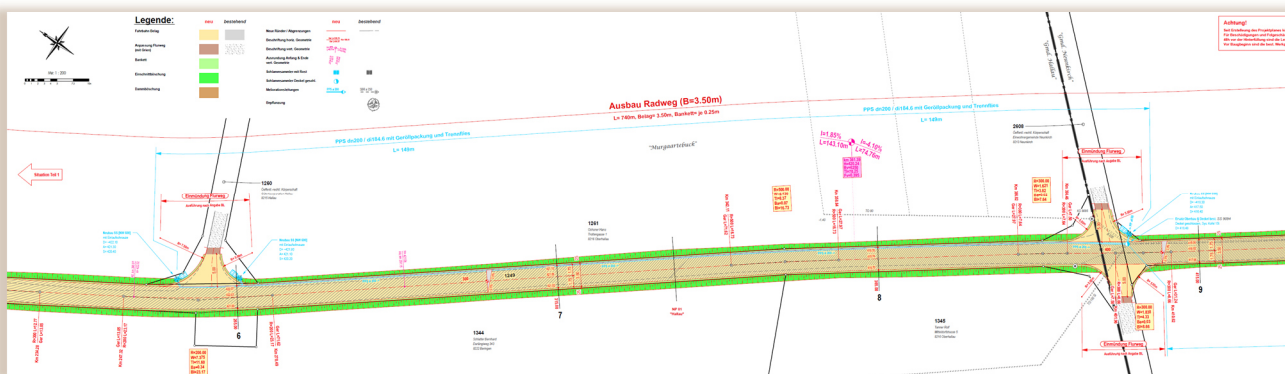
Normalprofil 01 "Hallau" 1:50
